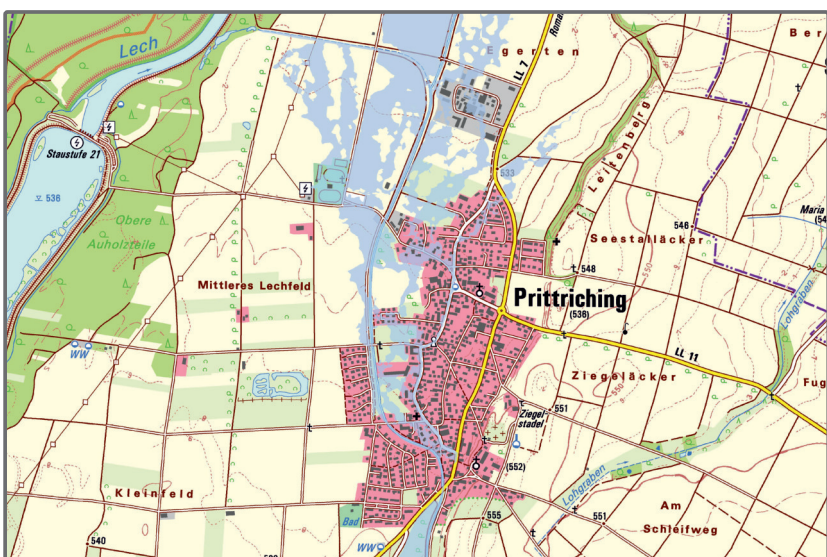
Überschwemmungsgebiet (Ist-Zustand) Vorläufig gesichertes Überschwemmungsgebiet
